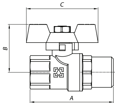
Кран кульовий з метеликом серії Yellow (3P-BP)
