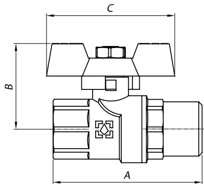
Кран шаровой с бабочкой серии Yellow (BP-HP)
