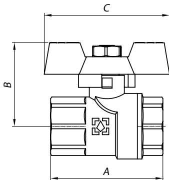
Кран кульовий з метеликом серії Yellow (BP-BP)
