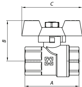
Кран шаровой с бабочкой серии Yellow (BP-BP)
