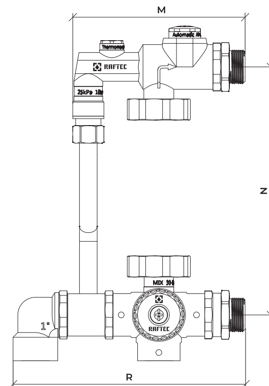
Габаритні розміри
