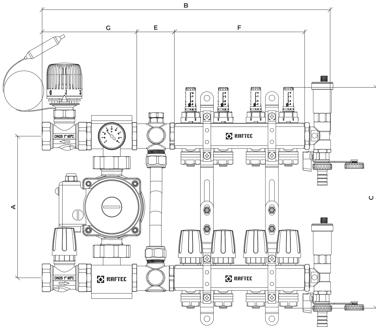
Габаритні розміри
