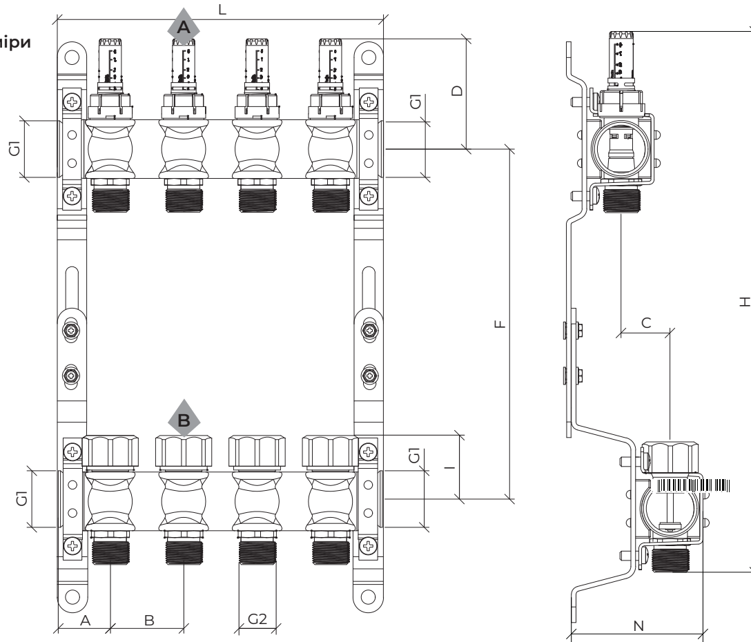
Колекторний блок з витратомірами RCO3
