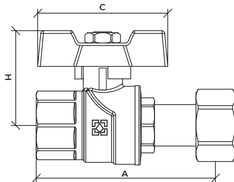
Kulový kohout s převlečnou maticí a vnitřním závitem série Black
