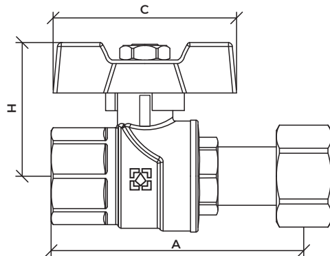
Кран шаровый прямой с накладной гайкой серии Black
