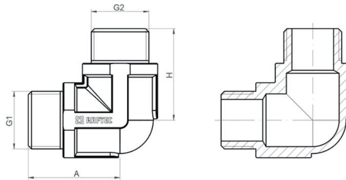
Кутник 90° ЗР-ЗР
