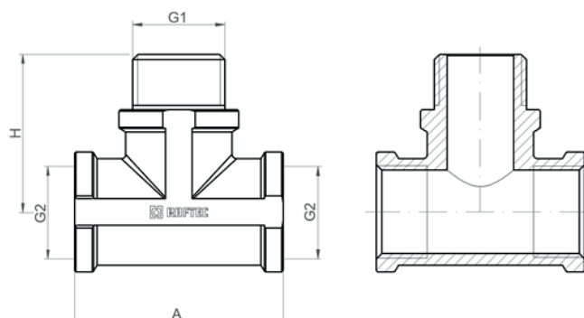
Трійник ВР-ЗР-ВР
