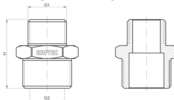
Ніпель перехідний ЗР-ЗР
