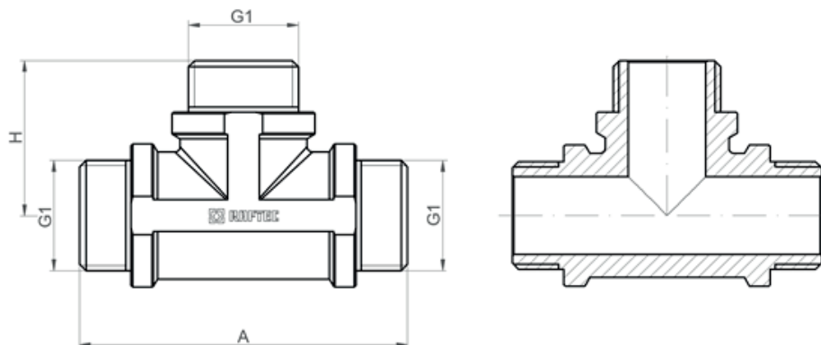
Трійник ЗР-ЗР-ЗР
