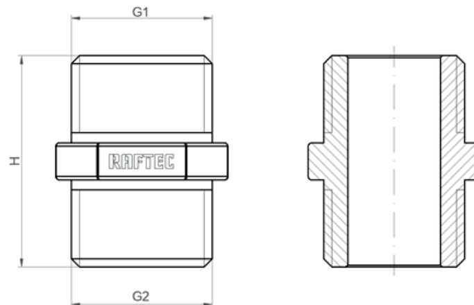
Ніпель ЗР-ЗР
