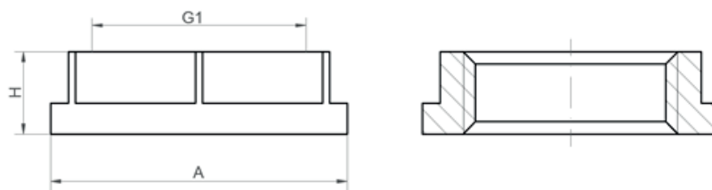
Контргайка ВР
