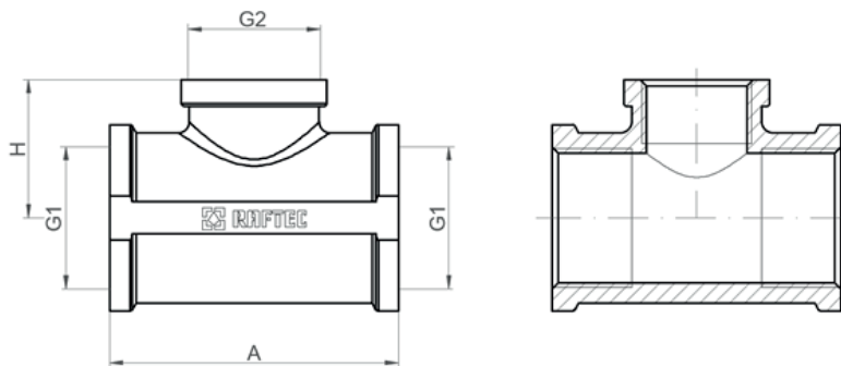
Трійник ВР-ВР-ВР
