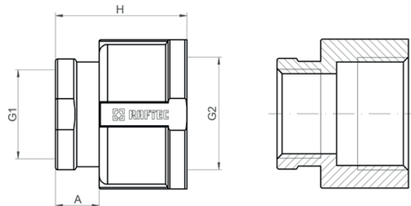
Муфта перехідна ВР-ВР
