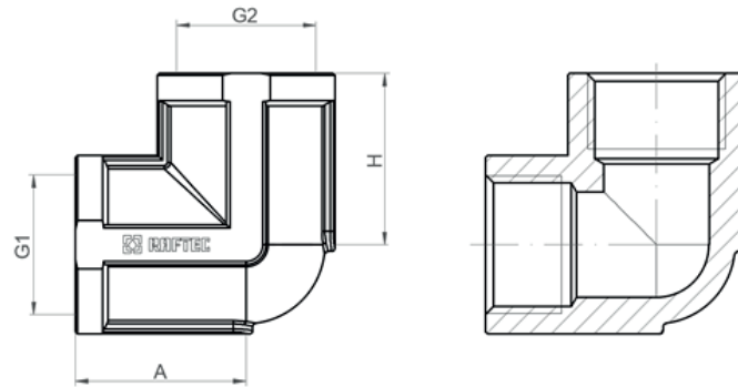
Кутник 90° ВР-ВР
