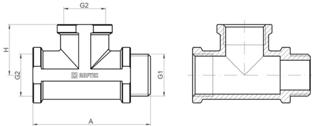
Трійник ВР-ВР-ЗР
