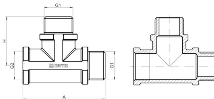
Трійник ВР-ЗР-ЗР
