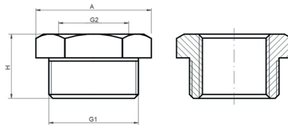
Футорка ВР-ЗР
