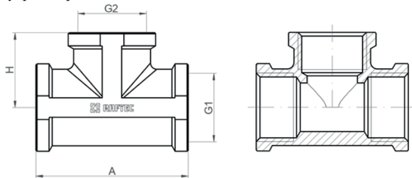
Трійник ВР-ВР-ВР
