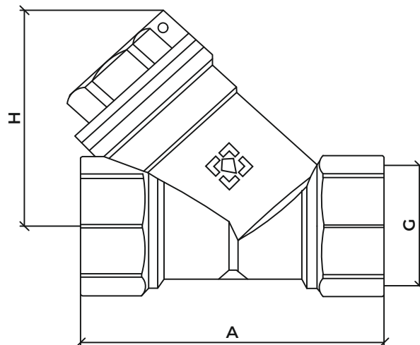
Фільтр механічного очищення ВР-ВР
